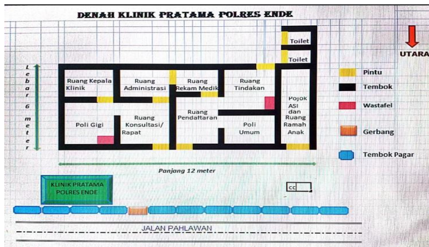
Gambar 1.4. Denah Klinik Pratama Polres Ende
